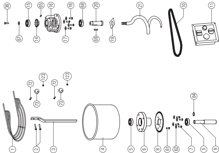
FIG. 19 Parti di ricambio impastatrice con testata e vasca fissa mod. IM 25-38-44 PICT. 19 Spare parts for mixer with fixed top and bowl mod. IM 25-38-44
