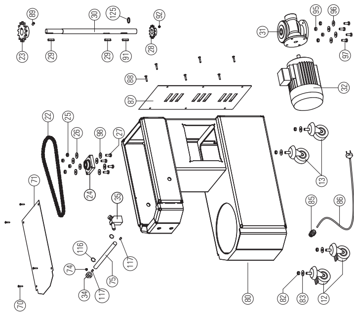
FIG. 19 Pièces de rechange pour pétrisseuse avec tête et cuve fixe mod. IM 25-38-44 BILD 19 Ersatzteile für die Teigmietmaschine mit gestern Kopf und Becken mod. IM 25-38-44
