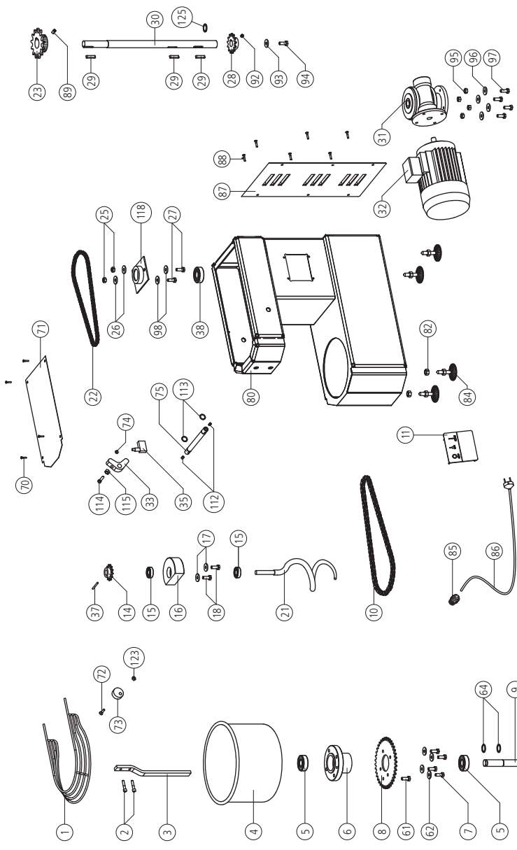
FIG. 17 Parti di ricambio impastatrice con testa e vasca fissa mod. IM 5-8 FIG. 17 Pièces de rechange pour pétrisseuse avec tête et cuve fixe mod. IM 5-8 PICT. 17 Spare parts for mixer with fixed top and bowl mod. IM 5-8 BILD 17 Ersatzteile für die Teigknetmaschine mit gestern Kopf und Becken mod. IM 5-8
