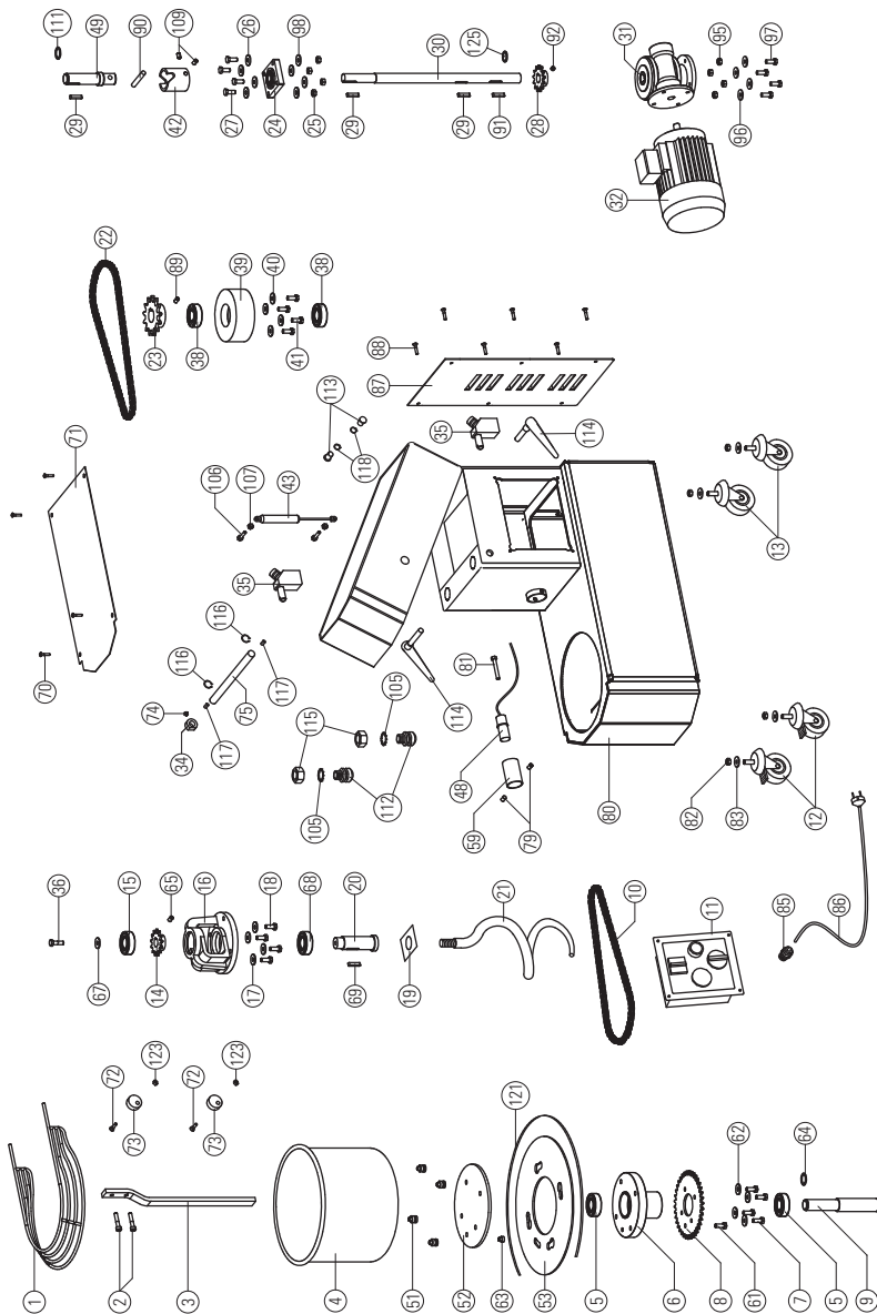
FIG. 22 Parti di ricambio impastatrice con testa sollevabile e vasca estraibile mod. IM 25-38-44 A FIG. 22 Pièces de rechange pour pétrisseuse avec tête soulevable et cuve extractible mod. IM 25-38-44 A PICT. 22 Spare parts for mixer with raising top and removable bowl. mod. IM 25-38-44 A BILD 22 Ersatzteile für die Teigknetmaschine mit hebbarem Kopf und herausziehbarem Becken mod. IM 25-38-44 A
